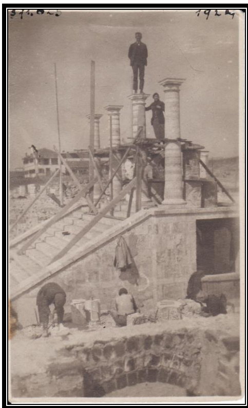
1924. Το χτίσιμο του Princeton Hall. Επάνω στην Κολόνα εικονίζεται ο κύριος Τσόουν Χένρυ Χάους με τους εργάτες να σφυρηλατούν τις ελαφρόπετρες στο σχήμα που απαιτείται και για την κατάλληλη θέση.
